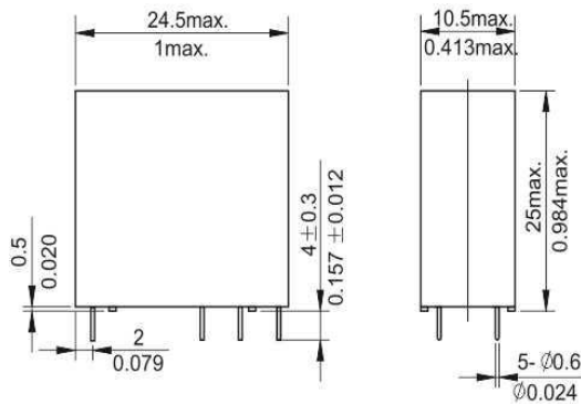
外形尺寸图 Dimensions
